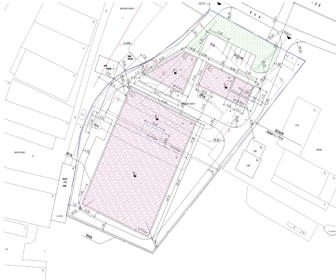
抚顺市盛益屠宰加工有限公司项目规划总平面图
