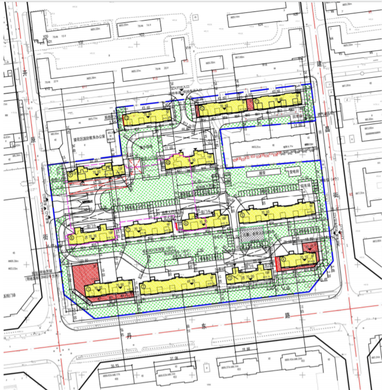
抚顺市百佳·新领域项目规划总平面图
