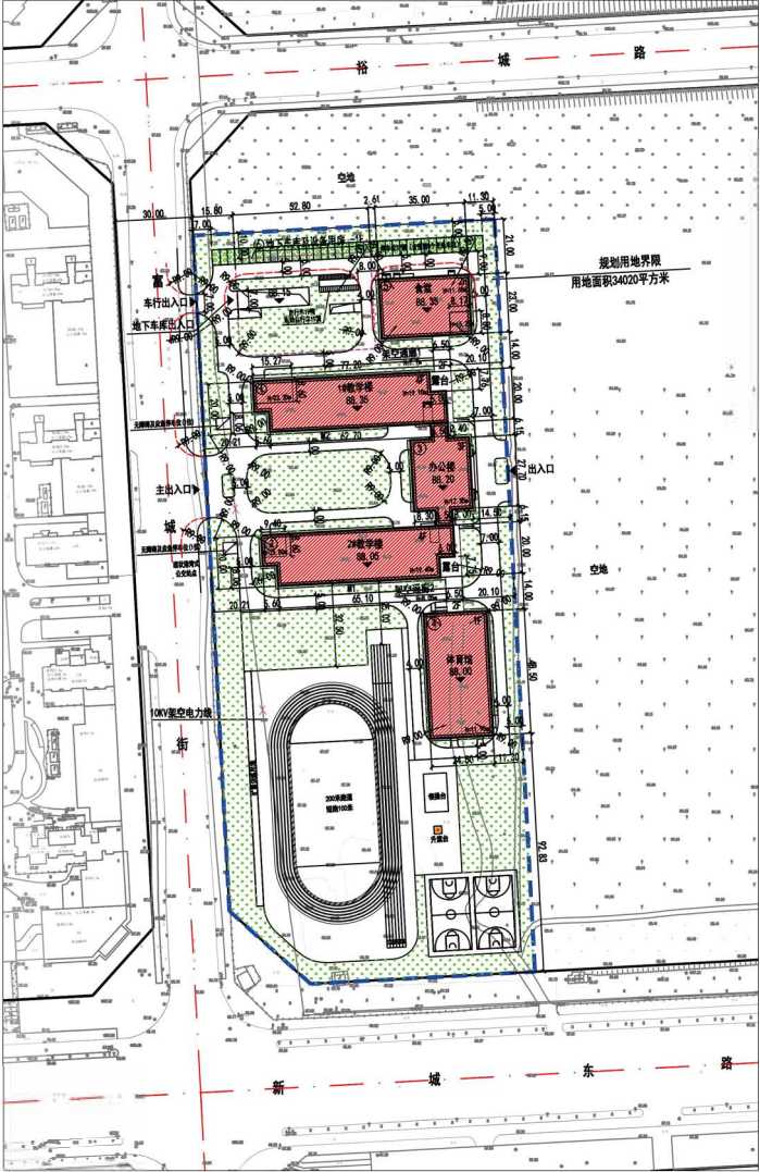
顺城区第三实验小学建设项目规划总平面图
