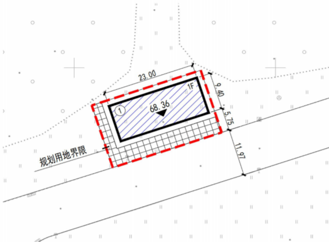
辽宁石油化工大学电力增容改造项目新建10KV开关站 规划总平面图
