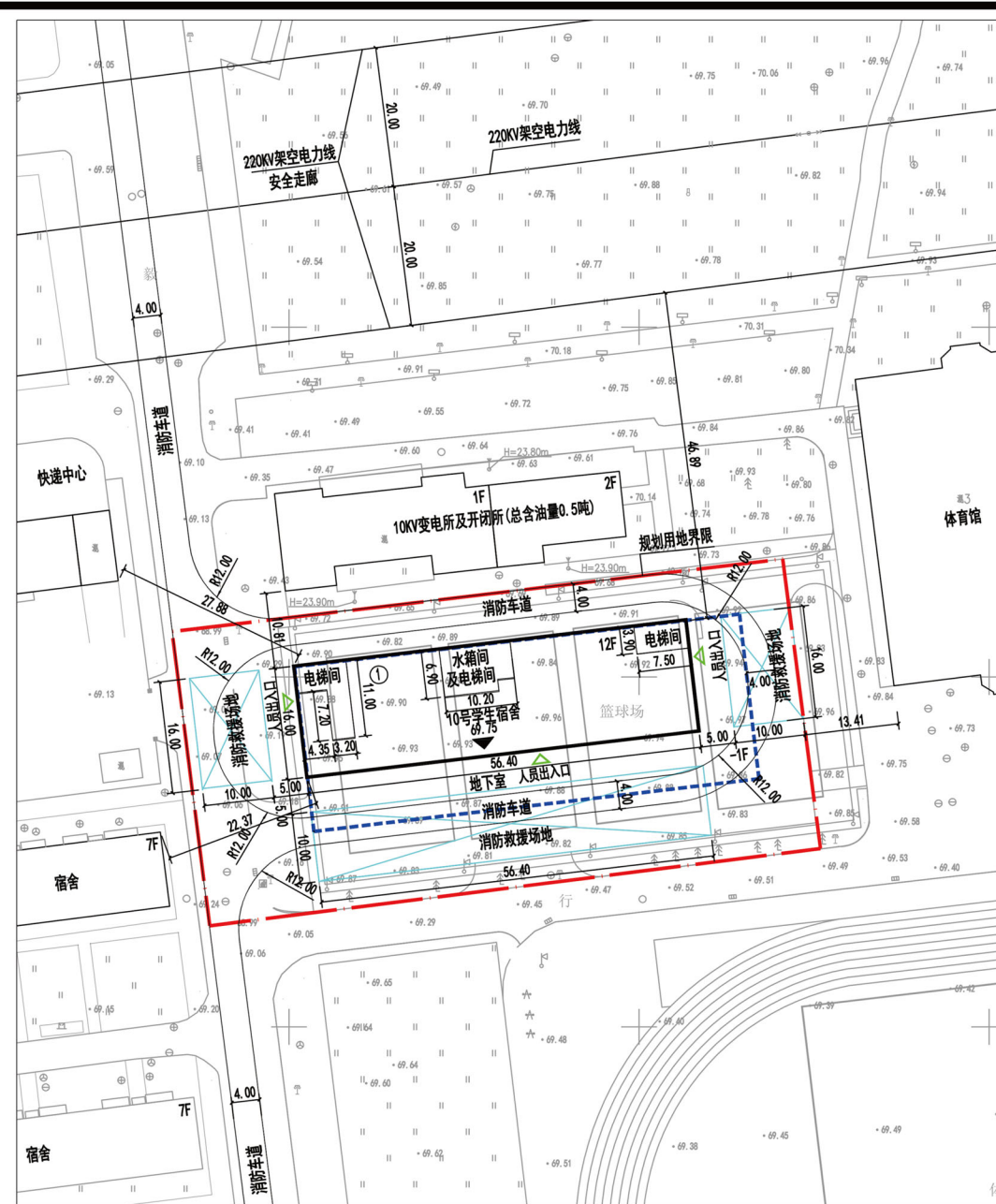
辽宁石油化工大学10号学生宿舍新建项目规划总平面图
