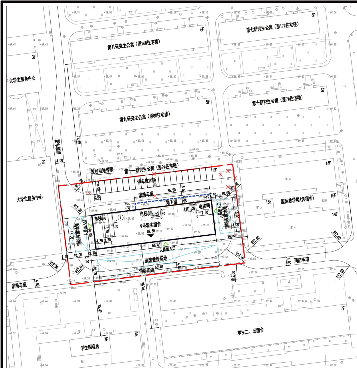
辽宁石油化工大学9号学生宿舍新建项目规划总平面图
