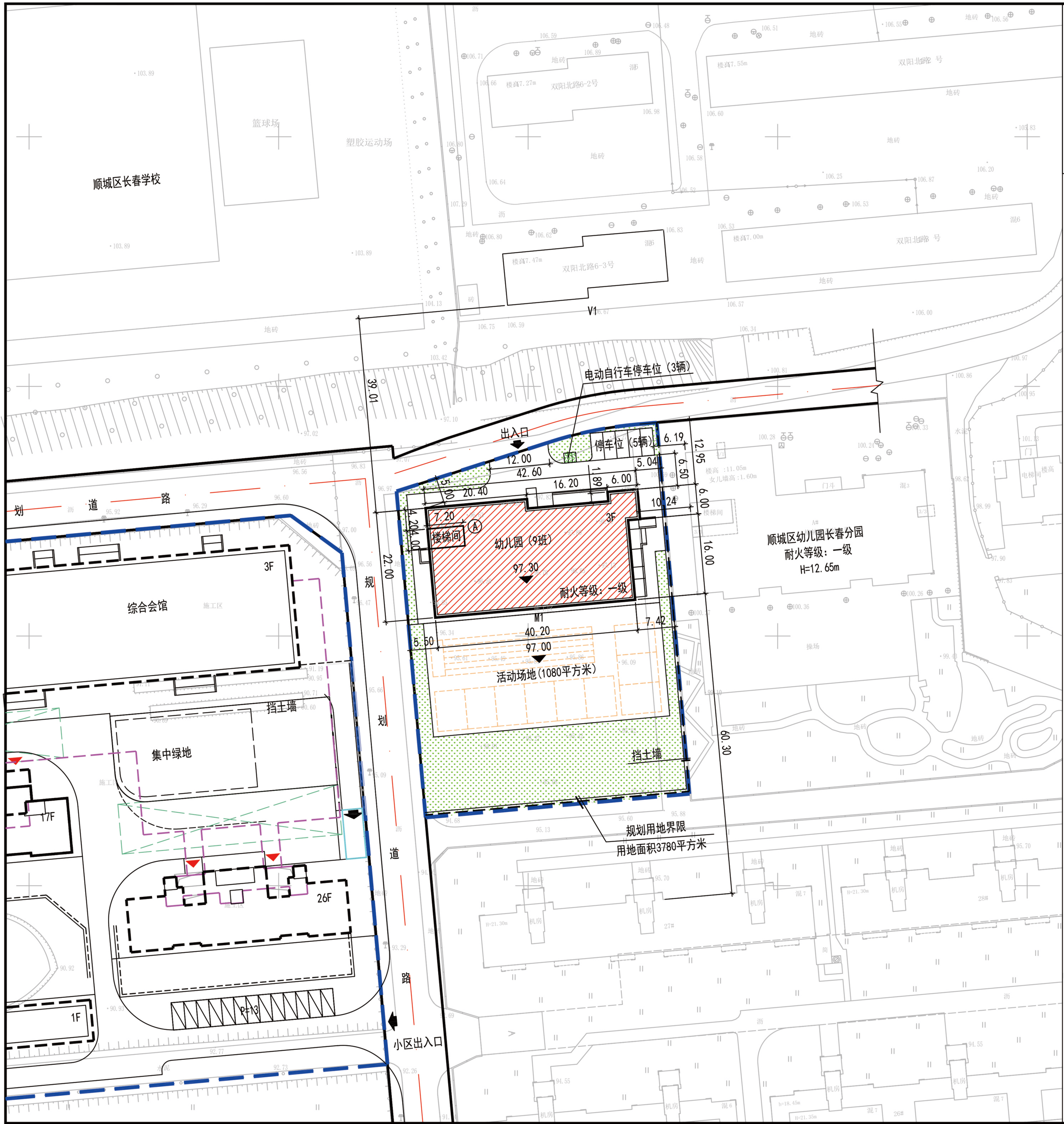
格林尚品三期幼儿园项目规划总平面图
