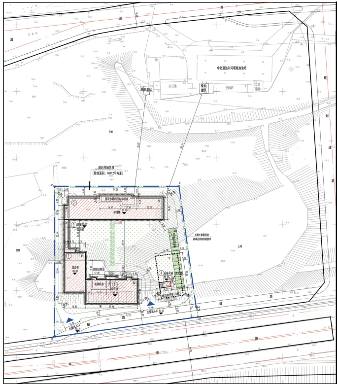
抚顺市新抚区公办养老福利中心新建项目规划总平面图
